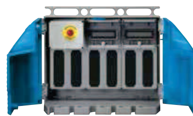
601532 € 342,00 Predisposto per 6 prese interbloccate (32A max) 9+9 moduli con pulsante emergenza frontale
